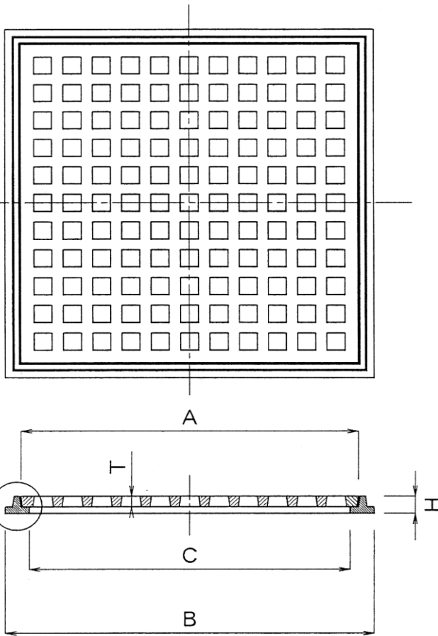
寸法・材質・表面处理・適応荷重
