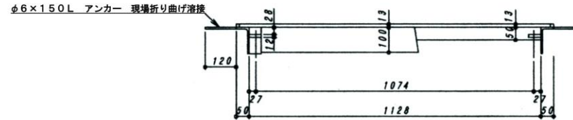
B-B断面図
