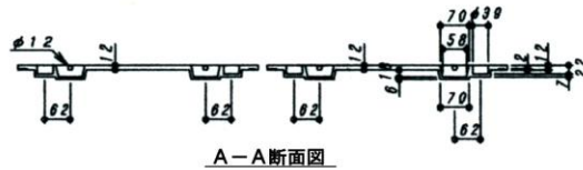
A-A断面図
