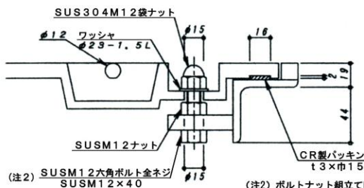
固定部詳細
