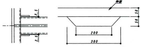
D部詳細
