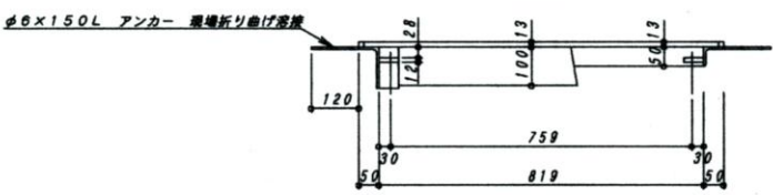
B-B断面図
