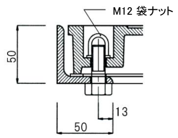
ネジ止め部詳細
