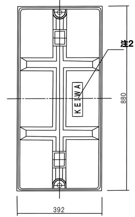
蓋裏面図
