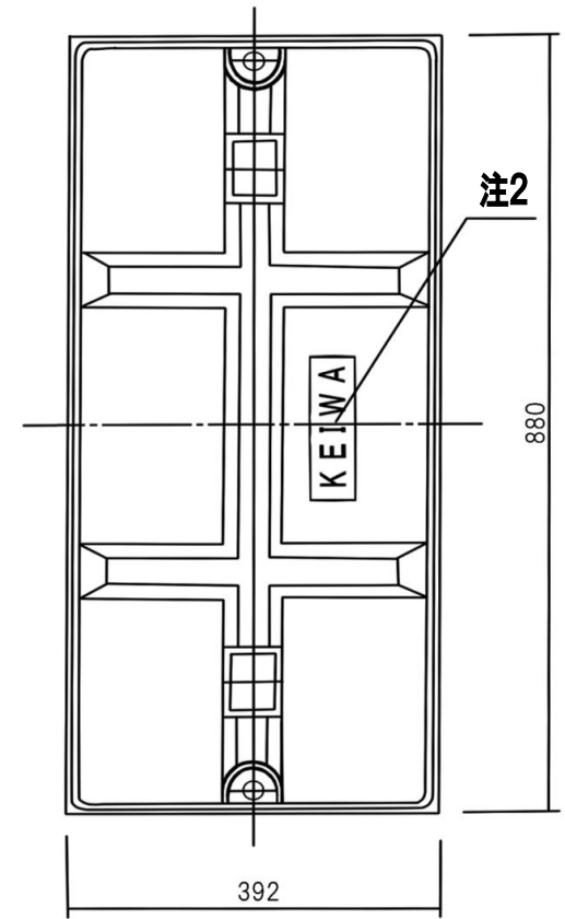
蓋裏面図
