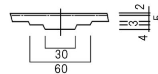
リブ部詳細
